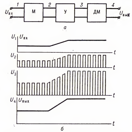
Рис. 3. Усилитель постоянного тока с преобразованием по частоте: а — схема; б — временные диаграммы напряжения сигнала в точках 1, 2, 3, 4; М — модулятор; У — бездрейфовый усилитель; ДМ — демодулятор; U вх — напряжение на входе; U вых — напряжение на выходе; U 1 , U 2 , U 3 , U 4 — напряжения в соответствующих точках усилителя; t — время.
